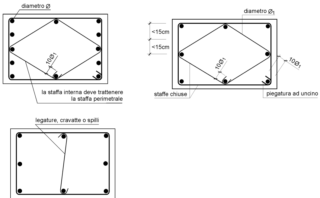
Fig. 1 - Indicazioni costruttive per strutture in calcestruzzo armato
