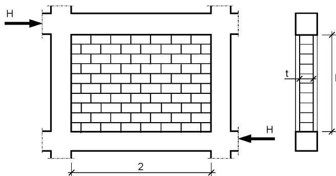
Fig. 2 - Interazione fra telai e pannelli murari di tamponatura
